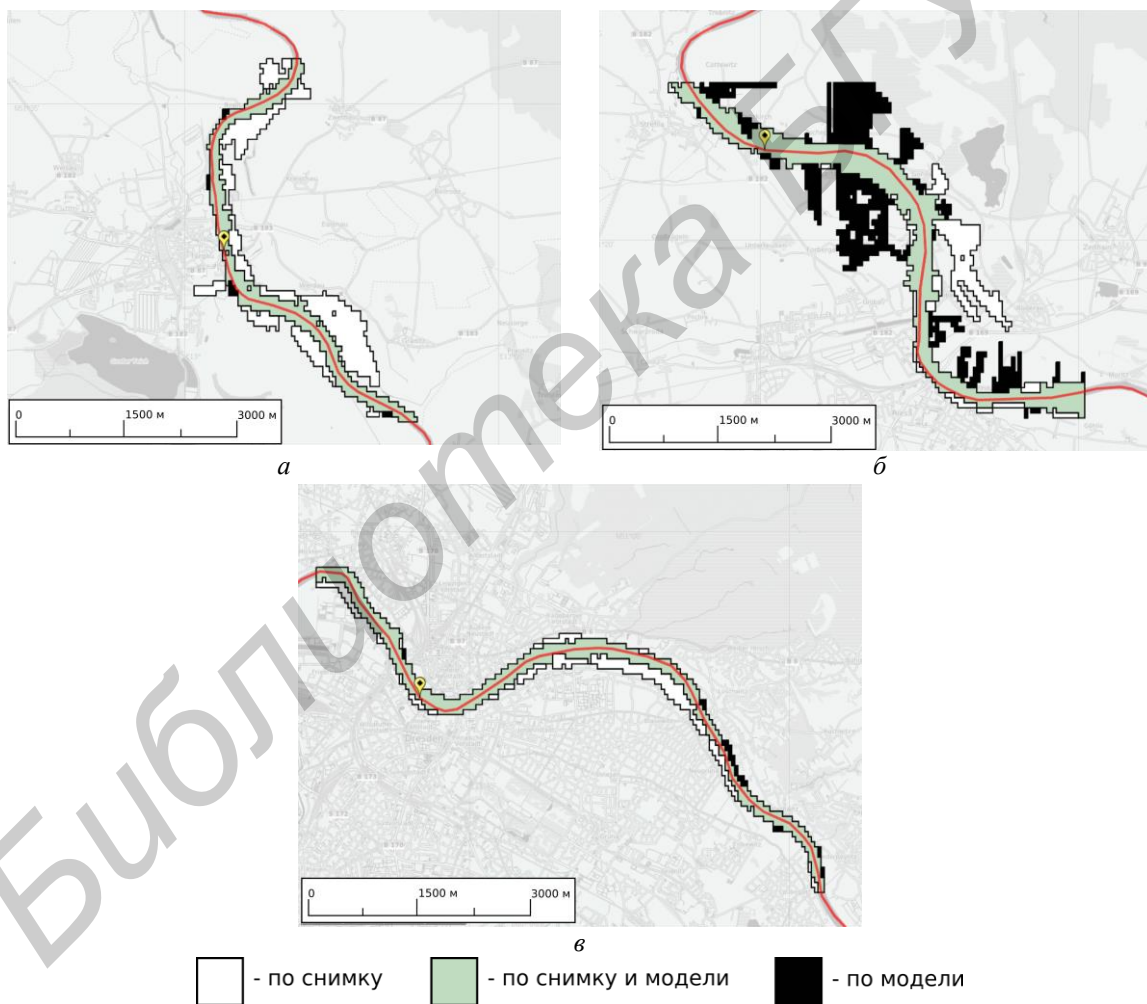
Рис. 4. Сравнение наблюдавшихся и вычисленных зон затопления с отметкой расположения ближайшего гидропоста: а – Торгау, б – Риза, в – Дрезден
