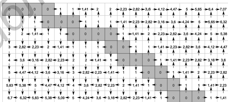
Рис. 2. Схема распространения фронта воды между ячейками ЦМР по градиенту кратчайшего Евклидова расстоянию от осевой линии реки
