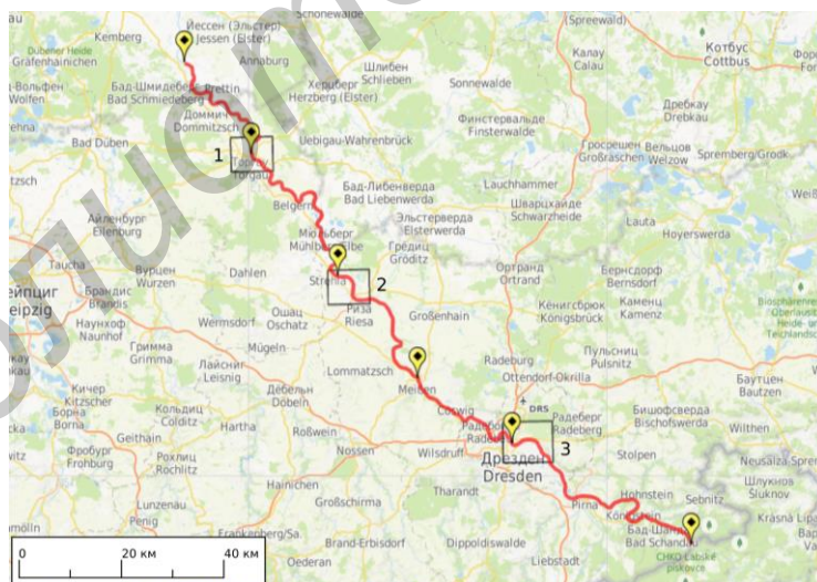
Рис. 3. Участок моделирования паводка на р. Эльба с расположением гидропостов; прямоугольниками отмечены районы проверки качества моделирования в окрестностях городов Торгау (1), Риза (2) и Дрезден (3).
