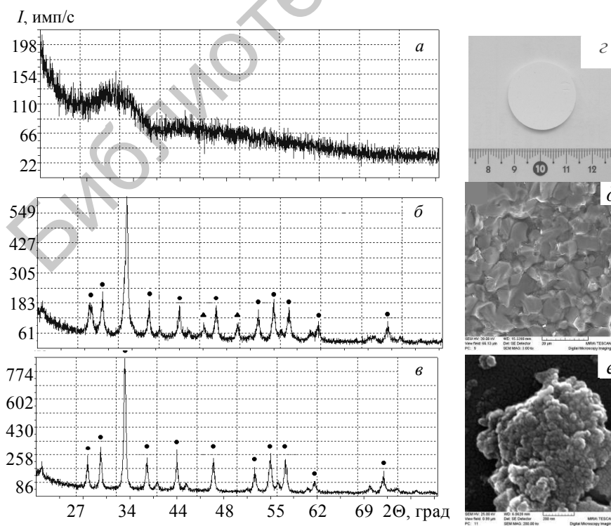
Рис. 1. Рентгеновские дифрактограммы Се–Cr-содержащей керамики (а–е), фотография керамики (з) и микрофотографии скола (д) и используемого для прессования порошка (е), T_{\text{отж}} = 800 (а, е), 900 (б), 1450^\circ\text{C} (в–д); рефлексы \text{Y}_3\text{Al}_5\text{O}_{12} (●) и \text{YAlO}_3 (▲)
